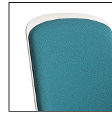
Schienale imbottito
